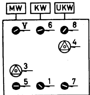
AM-Spulensatz von unten gesehen
